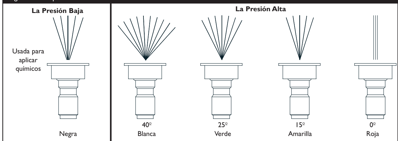
Figura 24 - Boquillas
